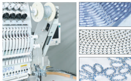
Zigzag Kordovací aparát
